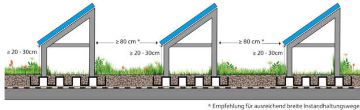
Abb. 10: Solargründach mit geneigten PV-Modulen in Süd-Ausrichtung. Quelle: BuGG
